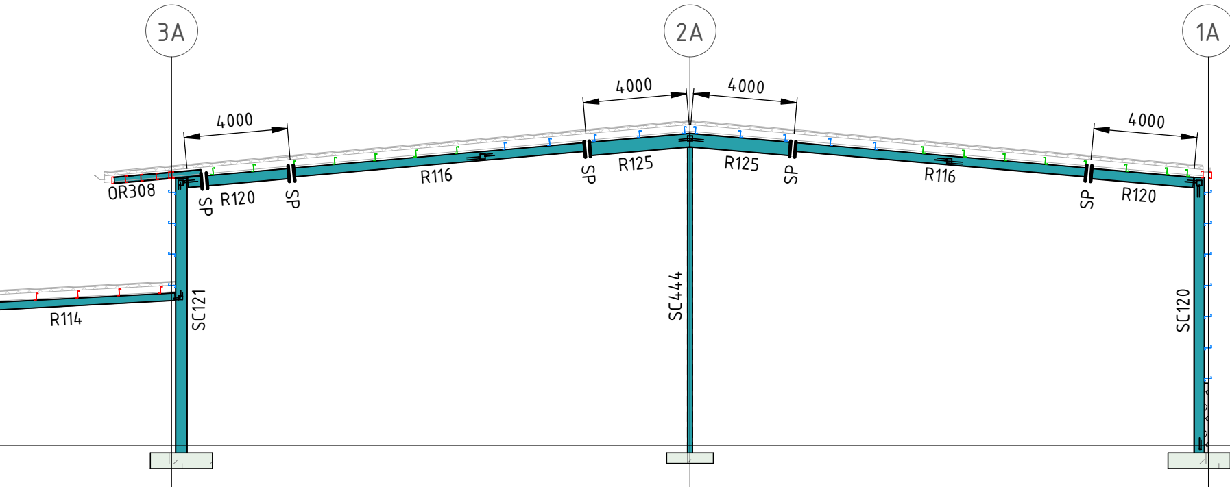
SECTION A7 SCALE 1 : 200
